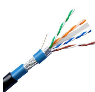
室外超六类铝箔+编织 双屏蔽网线 Outdoor SFTP Cat6
