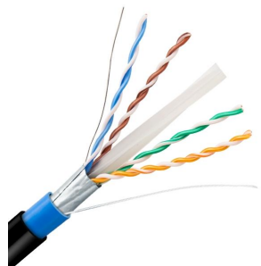
室外超六类铝箔屏蔽网线 Outdoor FTP Cat6
