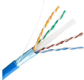
室内超六类铝箔屏蔽网线 Indoor FTP Cat6
